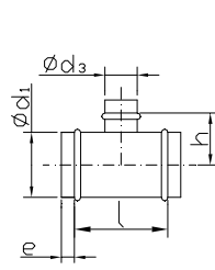
Pravokotni T-kos - TKP
