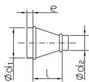
Reducirni sredinski kos - RSK
