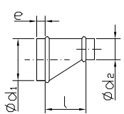
Reducirni zamačni kos - RZK
