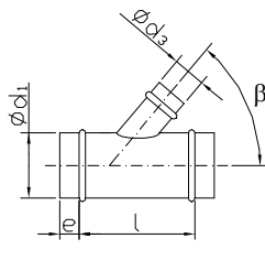
T-kos pod kotom - TKK
