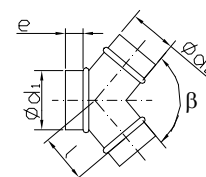
Razvodni Y-kos - RY
