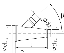
Reducirni T-kos pod kotom - RTKK
