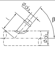
Sedlasti nastavek pod kotom - SNK
