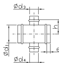
Križni X-kos - KX
